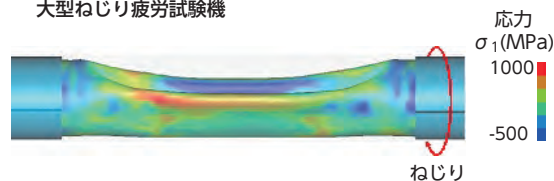
鋼管のねじり変形数値解析
