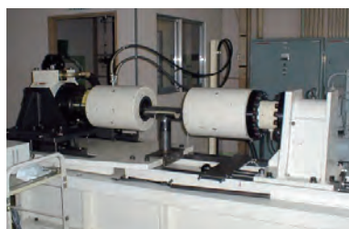
大型ねじり疲労試験機
